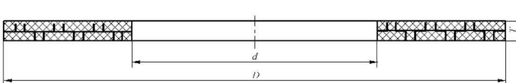
图 2 带螺栓孔型垫片结构型式
